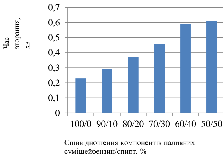
Рис.9. Залежність часу згорання бензиново-етанольної суміші (хв) в залежності від частки абсолютного етанолу
