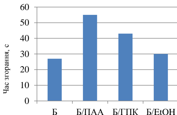
Рис.8. Залежність часу згорання від природи доданого активатора згорання (5% мас.): (Б-бензин А-92, Б/ПАА-суміш бензину та параацетальдегіду, Б/ГПК-суміш бензину та кумол гідропероксиду, Б/EtOH-суміш бензину та етилового спирту).
